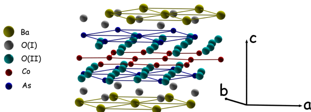
FIG. D.1: Structure cristallographique de BaCo_2(AsO_4)_2 . Succession des différentes couches selon l'axe c : Ba , O1 , As , O2 , Co , O2 , As , O1 , Ba . Le réseau d'ions cobalt est imbriqué entre deux plans compacts de tétraèdres AsO_4 .
