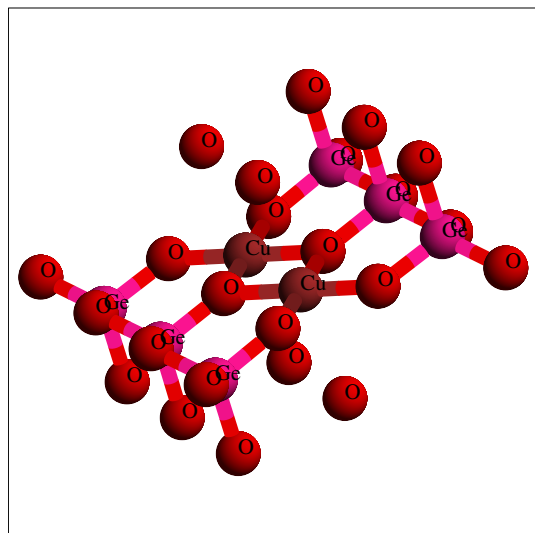
Dimère de cuivre dans CuGeO_3 .
