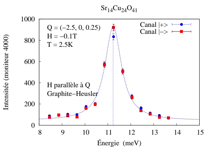
FIG. E.34: Spectre inélastique dans les chaînes mesuré en champ nul. Le faisceau incident est non polarisé. Le champ magnétique faible -0.1T est appliqué dans la direction du vecteur de diffusion Q pour permettre l'analyse de l'état de polarisation du faisceau diffusé parallèlement à Q .
