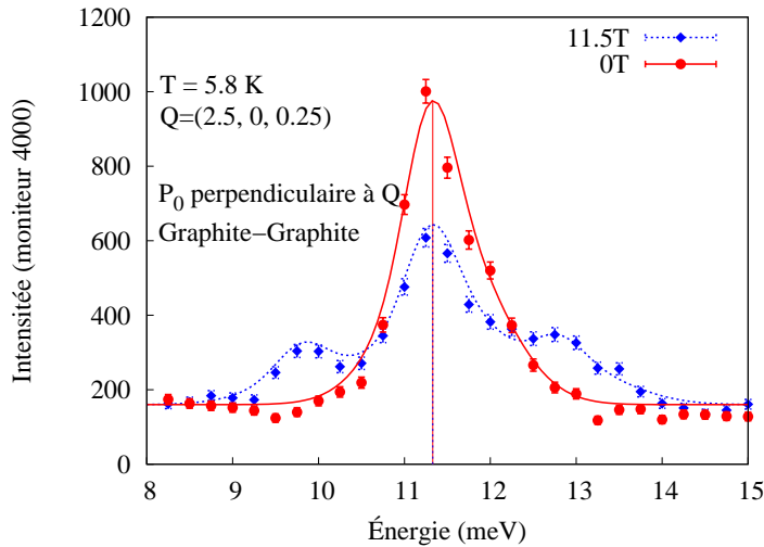
FIG. E.33: Spectre inélastique dans les chaînes mesuré avec des neutrons non polarisés en champ nul et sous 11.5T vertical, à basse température.
