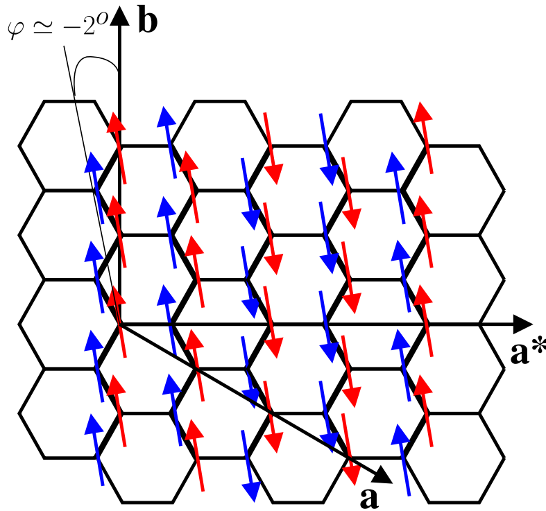
FIG. D.21: Représentation de la structure magnétique dans le plan (\mathbf{a}, \mathbf{b}) pour le modèle pseudo-colinéaire avec comme hypothèse que le vecteur de propagation de la structure est commensurable ( k_{0x} \simeq 1/4 ), que le déphasage \Phi^{ab} est presque 90^\circ avec l'origine \Phi_1^{ab} égale à \frac{\pi}{4} ou -\frac{\pi}{4} .
