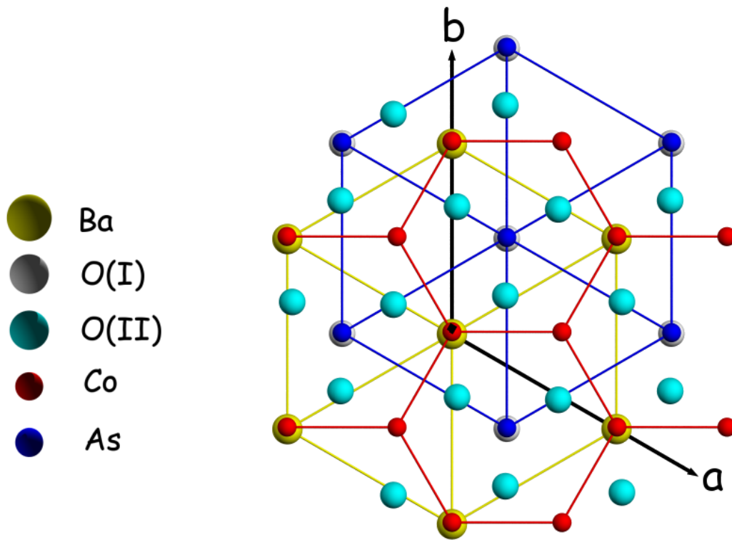
FIG. D.3: Projection selon l'axe c des différentes couches. En rouge le réseau en nid d'abeille des ions Co^{2+} , en bleu le réseau trigonal des ions As , chaque ion As est situé au centre d'un hexagone de cobalt. En jaune le réseau trigonal d'ion Ba . Chaque ion Ba est à l'apogée d'un ion Co^{2+}
