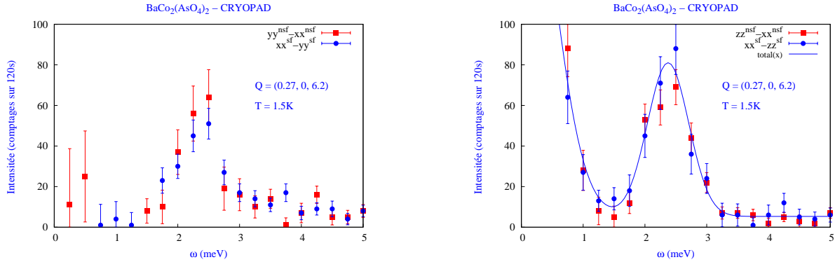
(a) Mesure de \sigma_M^y \approx \sigma_x^{sf} - \sigma_y^{sf} \equiv \sigma_y^{nsf} - \sigma_x^{nsf} au vecteur \mathbf{Q}=(0.27,0,6.2) sur une gamme d'énergie allant de 1 à 5 meV. (b) Mesure de \sigma_M^z \approx \sigma_x^{sf} - \sigma_z^{sf} \equiv \sigma_z^{nsf} - \sigma_x^{nsf} au vecteur \mathbf{Q}=(0.27,0,6.2) sur une gamme d'énergie allant de 1 à 5 meV.
