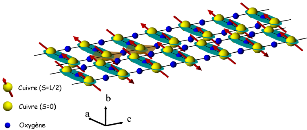
FIG. E.8: Représentation tridimensionnelle du système de dimères de spins dans les échelles à deux montants du composé pur Sr_{14}Cu_{24}O_{41} . On peut voir sur cette figure une représentation de l'échange anti-ferromagnétique isotrope entre les montants et les barreaux d'une échelle. La frustration magnétique est nettement visible entre deux échelles. L'environnement de champ cristallin de l'ion cuivre Cu^{2+} dans les échelles et aussi de type plan-carré mais ce dernier est de plus grande étendue spatiale que dans les chaînes.
