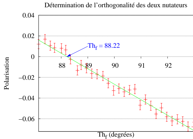
FIG. C.5: Première étape : le nutateur incident a pour consigne th_i = 0 , nous scanons le nutateur de sortie autour de la consigne th_f = 90^\circ en s'assurant qu'il n'y a aucun courant dans les bobines de précession. En l'absence de champ parasite, lorsque la polarisation s'annule, les deux nutateurs sont parfaitement orthogonaux.
