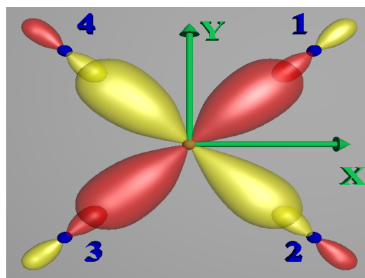
Orbitales d en géométrie plan carré. Les densités de probabilité rouges sont positives.
