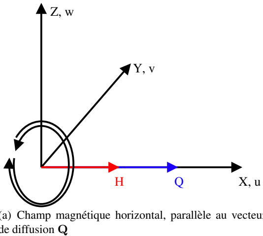
FIG. E.41: Configurations horizontale et verticale du champ magnétique par rapport au vecteur de diffusion \mathbf{Q} .
