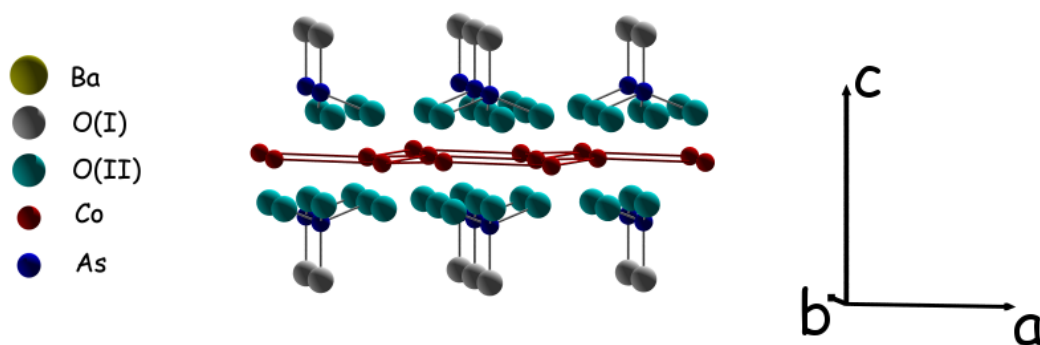
FIG. D.2: Le réseau en nid d'abeille d'ion Co^{2+} est imbriqué entre deux couches de type AsO_4 formant des tétraèdres indépendants les uns des autres, les tétraèdres pointent vers l'extérieur de la structure et sont tournés les uns par rapport aux autres de \frac{\pi}{3} .
