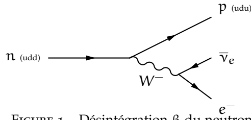
FIGURE 1 – Désintégration \beta du neutron
